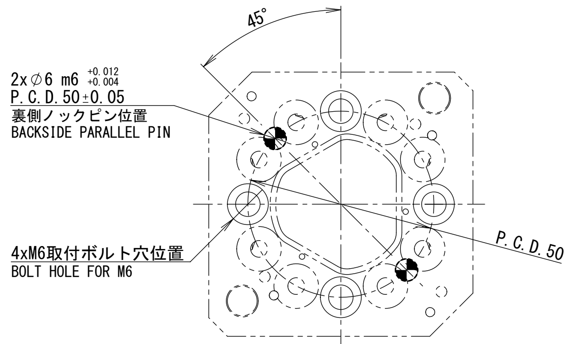
矢視図 A: 取合い寸法図 VIEW A: CONNECTING DIMENSION VIEW
