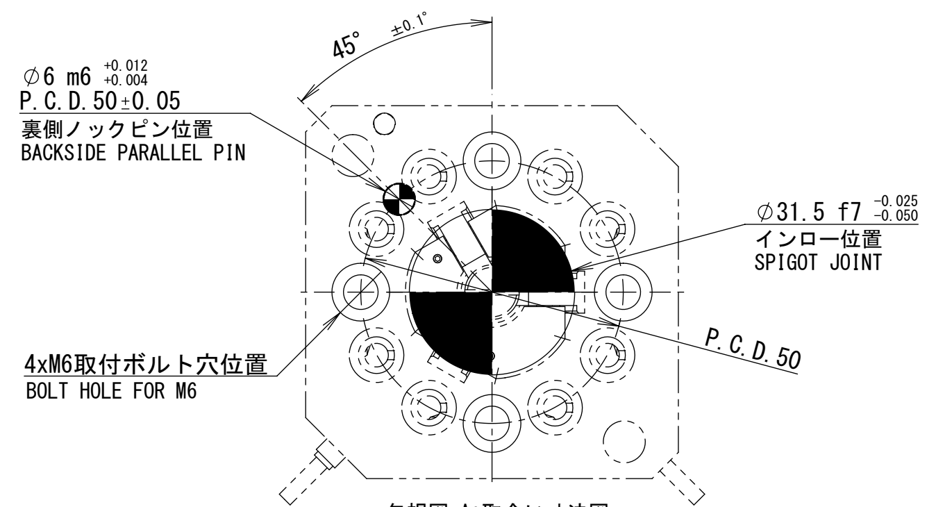
矢視図 A: 取合い寸法図 VIEW A: CONNECTING DIMENSION VIEW
