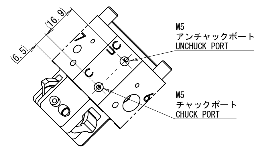
矢視図 B VIEW B
